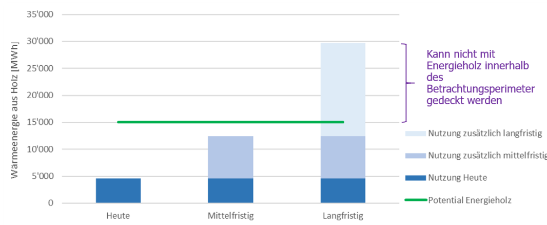
Abbildung 10: Gegenüberstellung Nutzung und Potential Energieholz zusammengefasst für alle 13 Gemeinden
