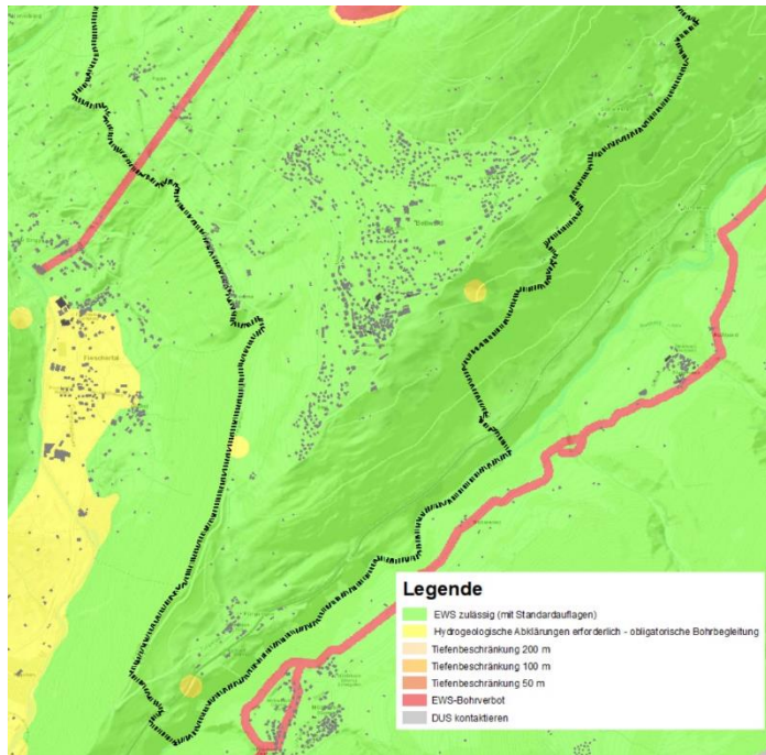
Abbildung 9: Zulässigkeitskarte für Erdwärmesondennutzungen im besiedelten Bereich von Bellwald.
