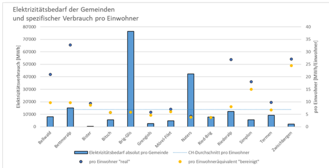
Abbildung 4: Übersicht Elektrizitätsbedarf (Balken) und pro Kopf Verbrauch der Gemeinden (Punkte).
