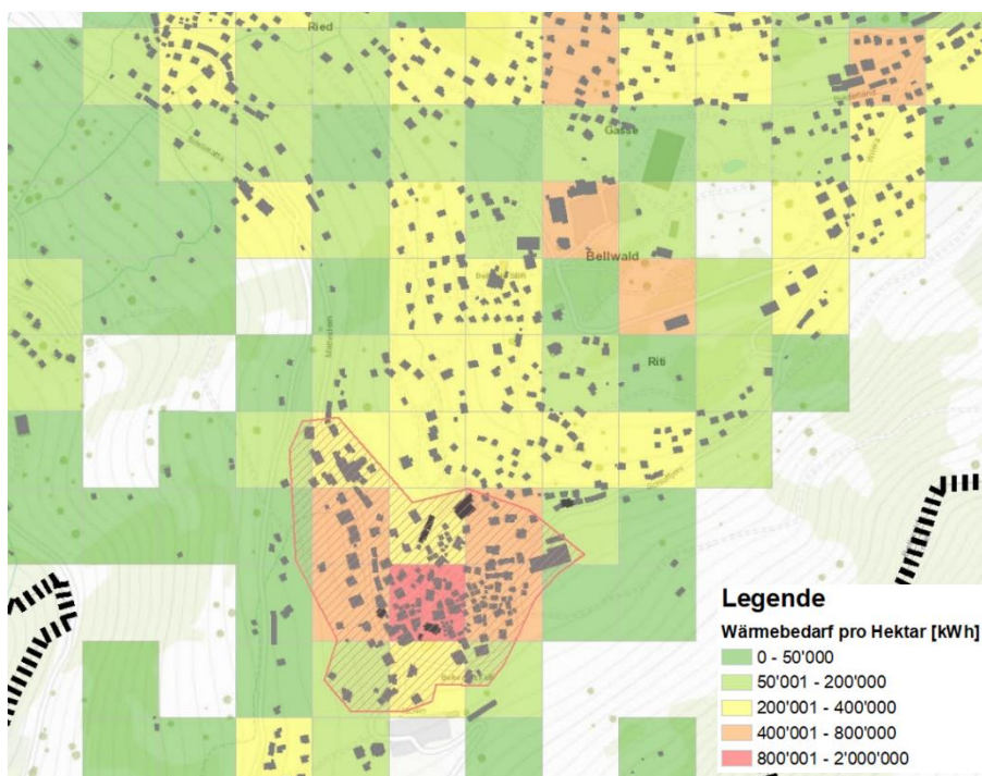
Abbildung 3: Wärmedichte im Hektarraster. Rot umrahmt das Gebiet, für welches eine Fernwärmeversorgung interessant sein könnte.
