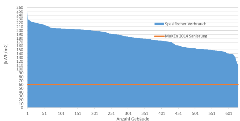
Abbildung 2: Spezifischer Wärmebedarf pro Gebäude in Bellwald in \text{kWh/m}^2\text{a} (blau) sowie der theoretische Verbrauch der mit einer Sanierung nach Energiegesetz erreichbar ist (orange). Auch wenn die Verbrauchsdaten zu hoch geschätzt wurden, geben die Angaben auf der Grafik ein Indiz, dass das Potential im Gebäudepark sehr hoch ist.
